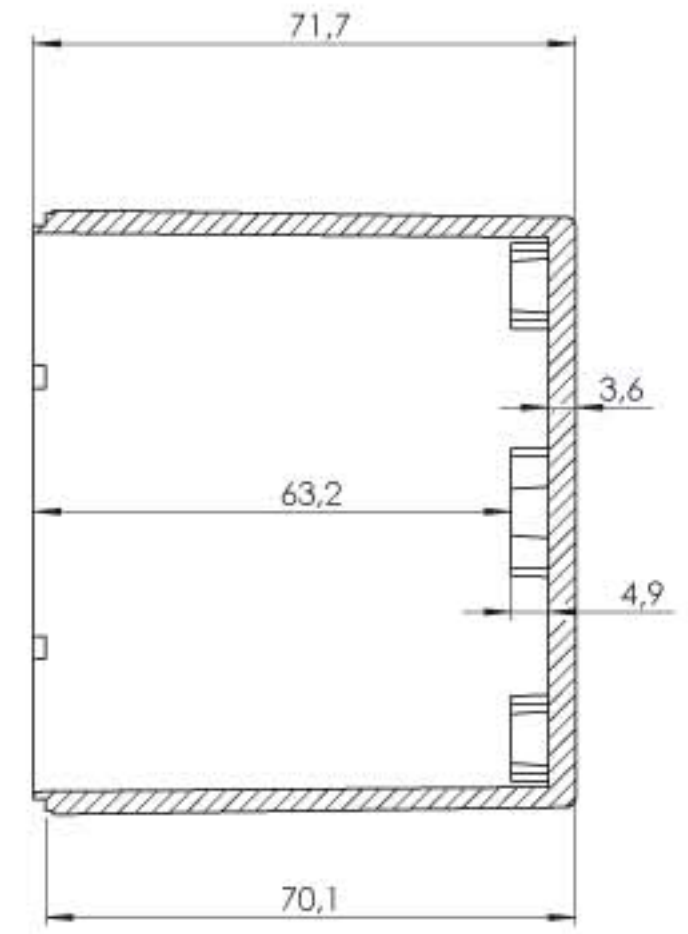
KESIT A-A
