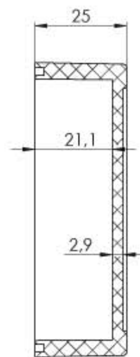
KESIT A-A
