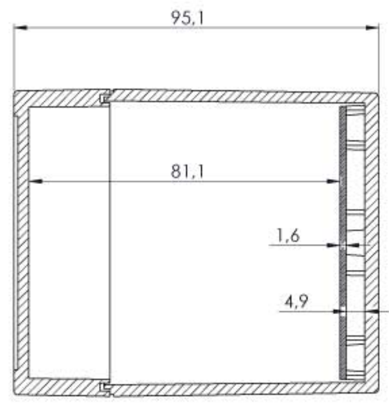
KESIT A-A
