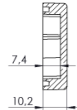
KESIT A-A
