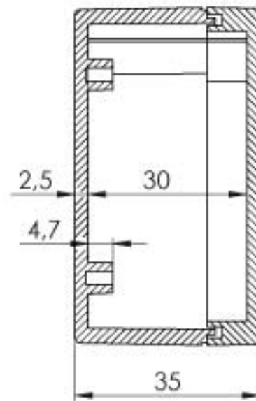
KESIT A-A
