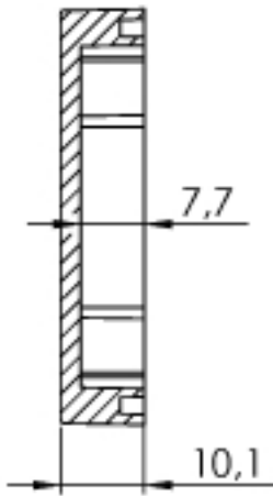
KESIT B-B
