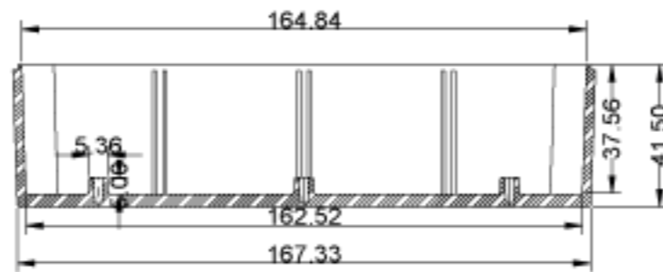
GOVDE KESITI
