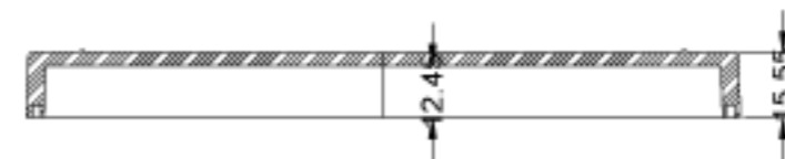
KAPAK KESITI
