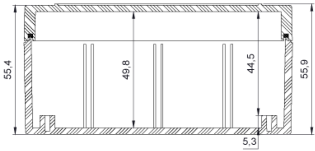
Kapak-Gövde Kesiti
