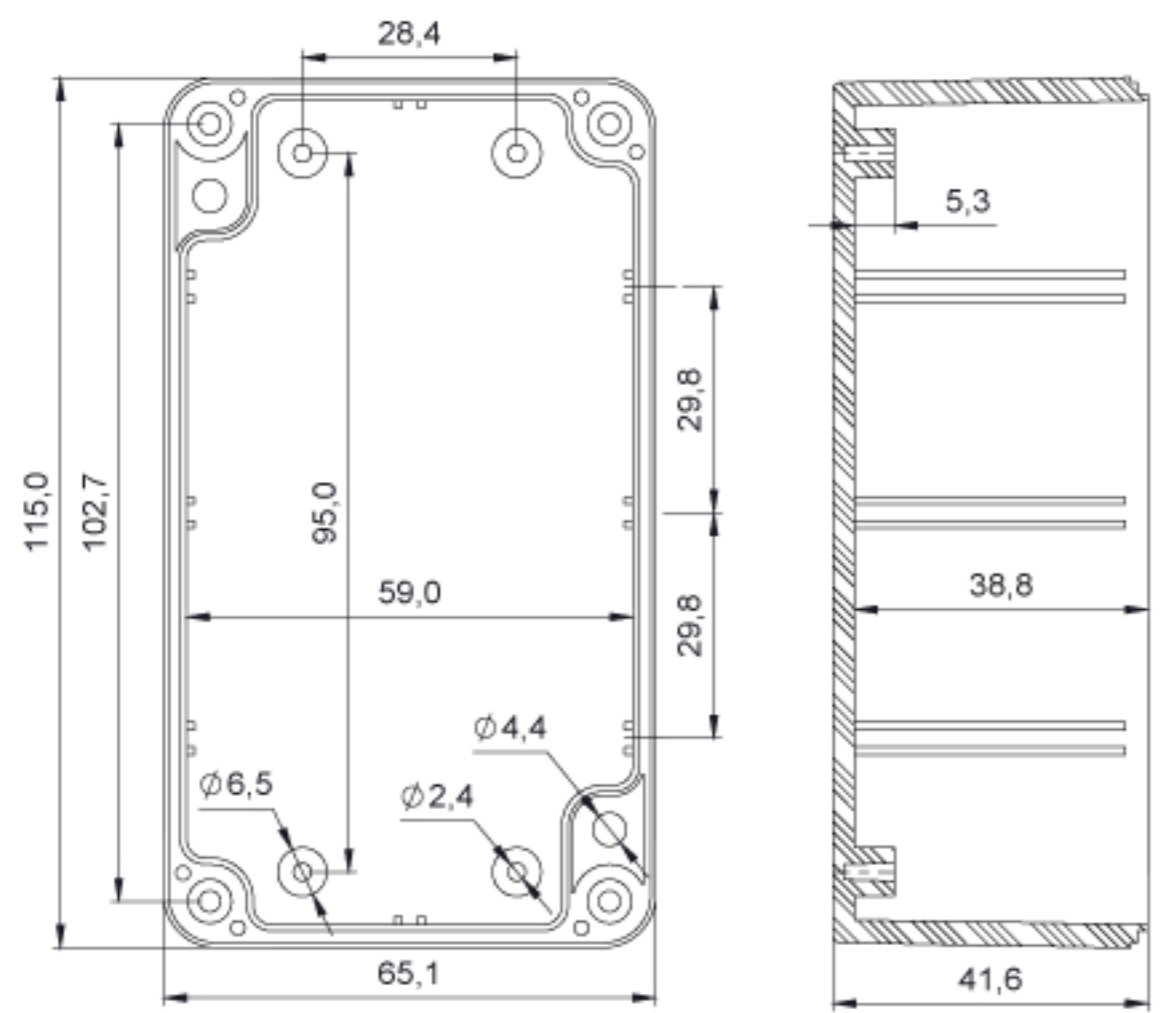
Gövde
