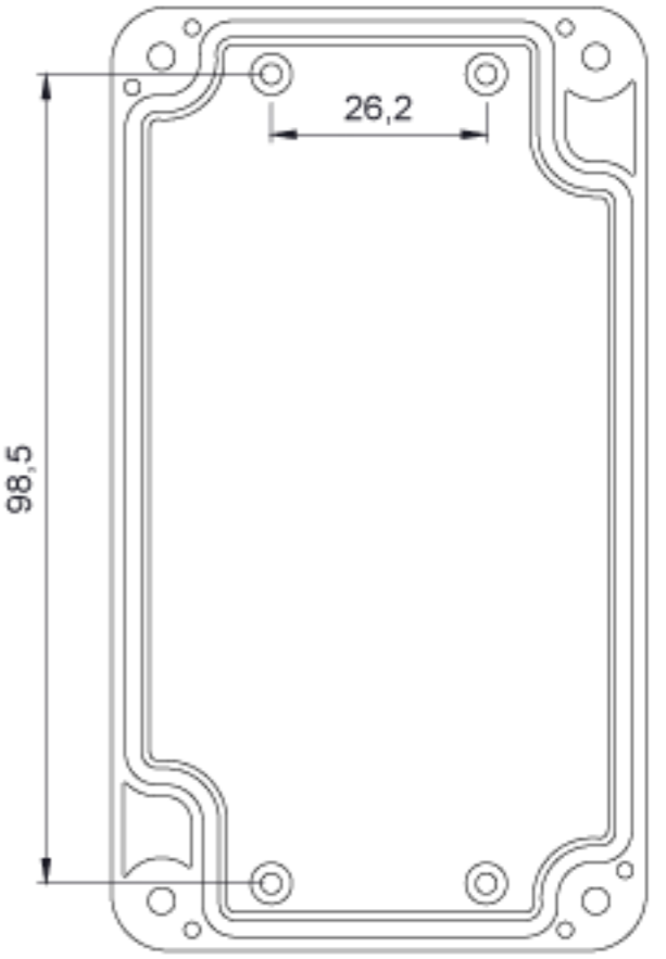
Kapak
