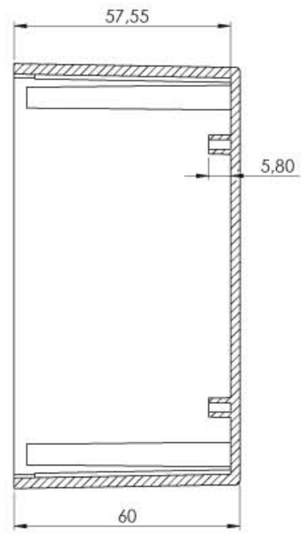
KESIT A-A
