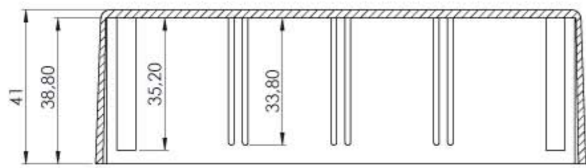
KESIT A-A
