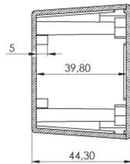
KESIT A-A
