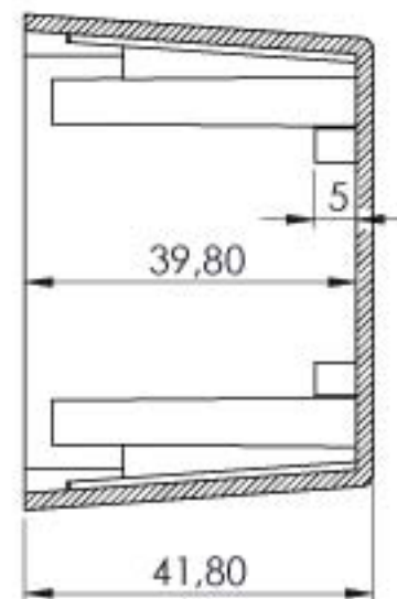
KESIT A-A
