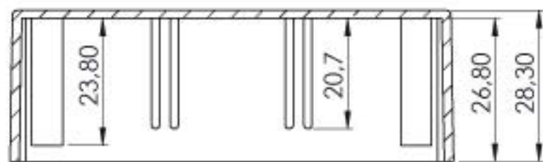
KESIT A-A
