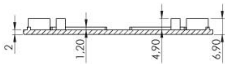
KESIT A-A
