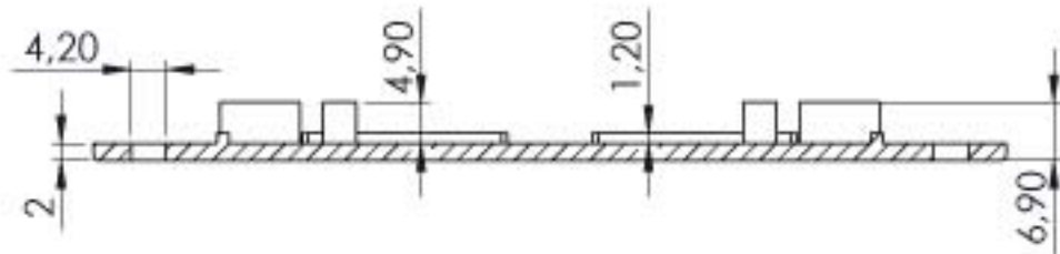
KESIT A-A
