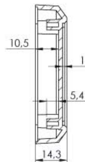
KESIT A-A
